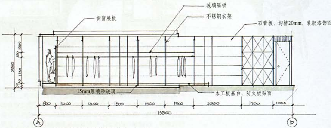
B向立面及天花剖面图 1:50
