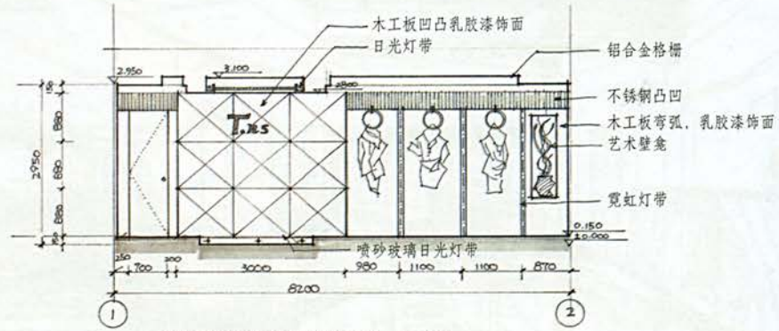
A向立面及天花剖面图 1:50
