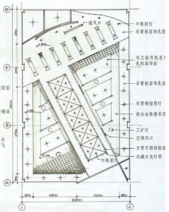
天花平面布局图 1:50
