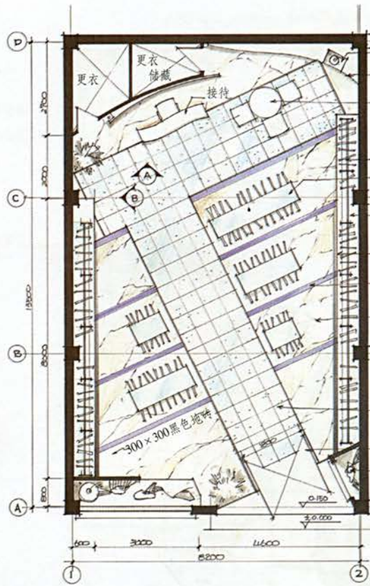
平面布局图 1:50
